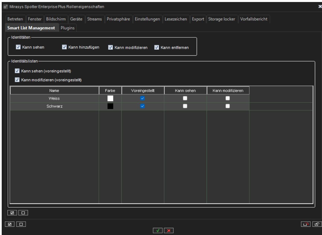
12 "Registerkarte "Intelligente Listenverwaltung"
